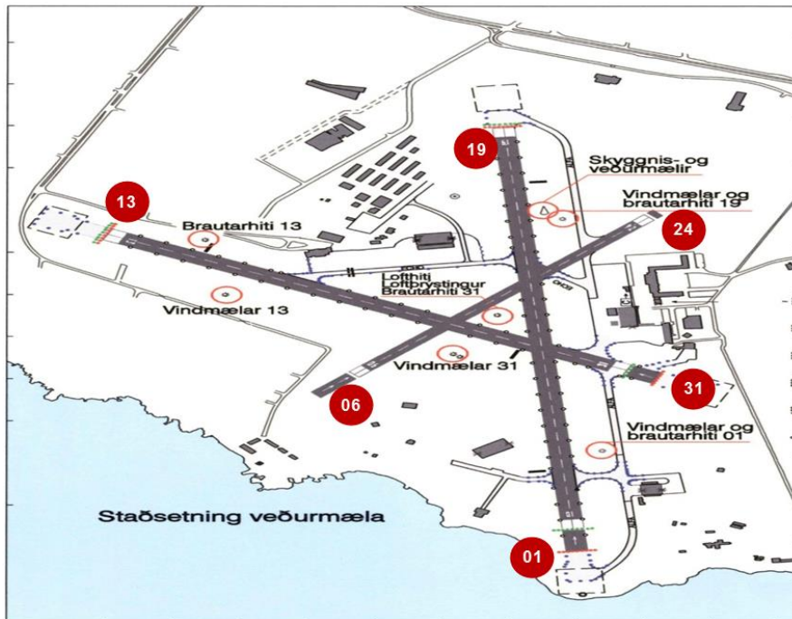
Mynd 1 Staðsetning vindhraðamæla og brautarnúmer.
